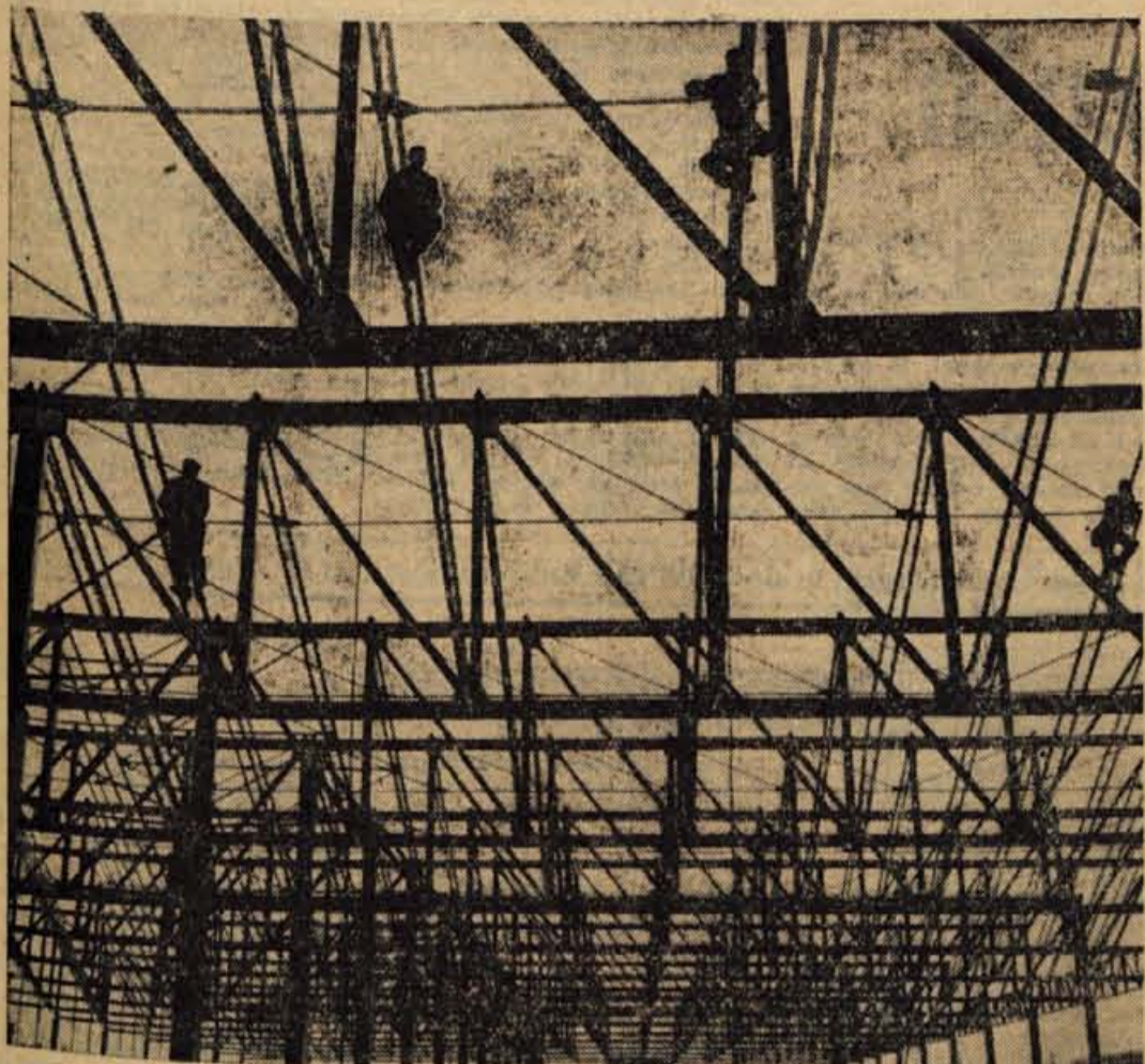
Ob obratu II kranjske tovarne gumijevih izdelkov Sava v Stražišču so zaključili z montažo jeklene konstrukcije hale za proizvodnjo tehničnega blaga. Predvidevajo, da bodo gradbena dela zaključena letos poleti. Proizvodna hala je dolga 160 metrov, široka pa 54 metrov. Ob njej bo dvonadstropni prizidek, kjer bodo sanitarije, garderobe, jedilnica, obratne pisarne in pomožni prostori proizvodnje. Gradbeni projekt je izdelalo podjetje »Slovenija-projekt«, izvedba jeklene konstrukcije je delo »Metalne Maribor, gradbena dela pa izvaja »Gradis« Ljubljana. Za jekleno konstrukcijo so porabili 320 ton jekla. Novi delovni prostori bodo delno namenjeni razširitvi proizvodnje, delno pa preselitvi nekaterih obratov iz obratov v centru mesta. — S.
