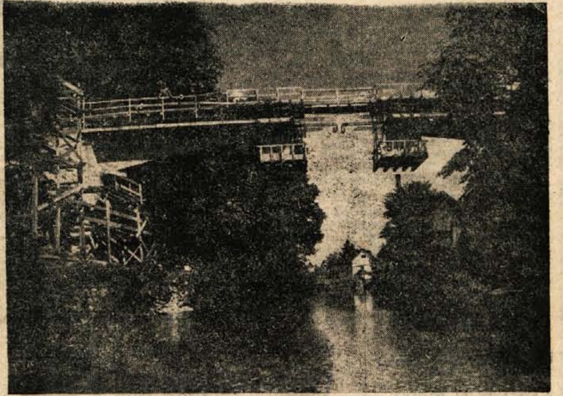
SGP Tehnik iz Skofje Loke se je prvo v Jugoslaviji lotilo nove gradnje mostu. Most čez Somo v Skofji Loki gradijo po delih - brže ko je določena dolžina betonskega mostu dovolj trdna, dograđijo spet nov del mostu (na sliki)
