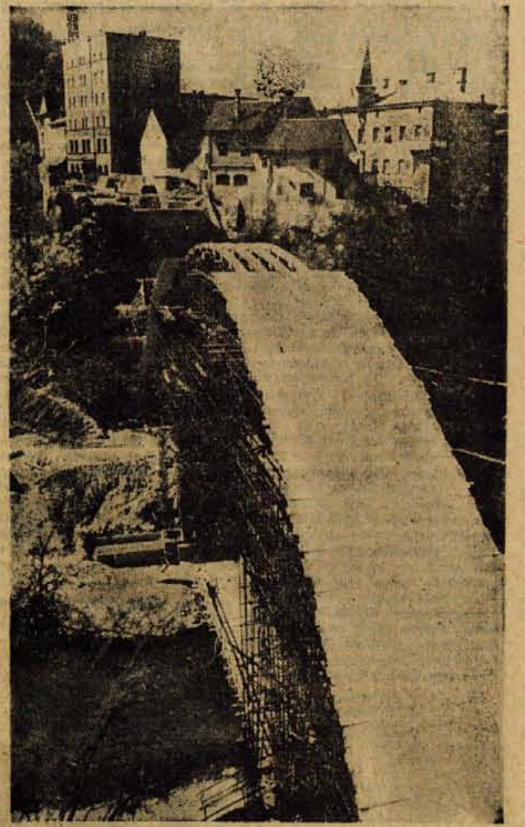
Približno pred enim mesecem smo v našem listu že objavili zanimivo sliko pomožne konstrukcije za novi most čez Kokro v Kranju. Vendar pa je bil takrat šele začetek gradnje, zato danes objavljamo novo sliko, ki prikazuje pomembno konstrukcijsko že skoraj povsem dograjeno
