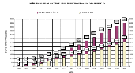
Rast hišnih priključkov na zemeljski plin v MO Kranj in občini Naklo
