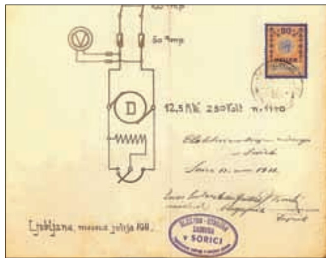
Del načrta soriške hidroelektrarne iz julija 1911, odobren 12. novembra 1911 od Elektro strojne zadruge v Sorici.
