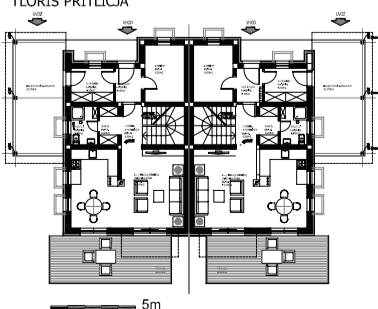
STANOVANJSKI DVOJČEK - OBJEKT C TLORIS PRITLIČJA
