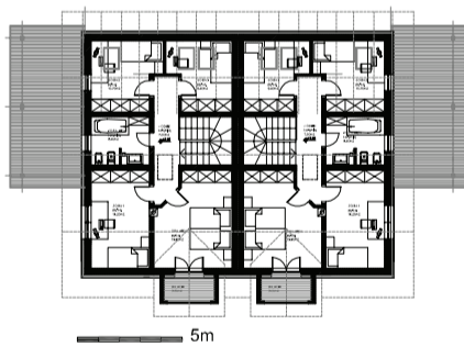
STANOVANJSKI DVOJČEK - OBJEKT B,D TLORIS MANSARDE
