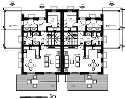
STANOVANJSKI DVOJČEK - OBJEKT B,D TLORIS PRITLIČJA
