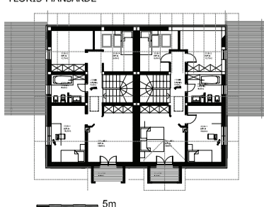
STANOVANJSKI DVOJČEK - OBJEKT C TLORIS MANSARDE
