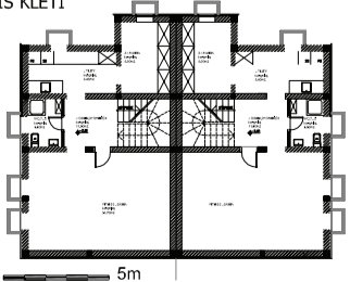
STANOVANJSKI DVOJČEK - OBJEKT C TLORIS KLETI
