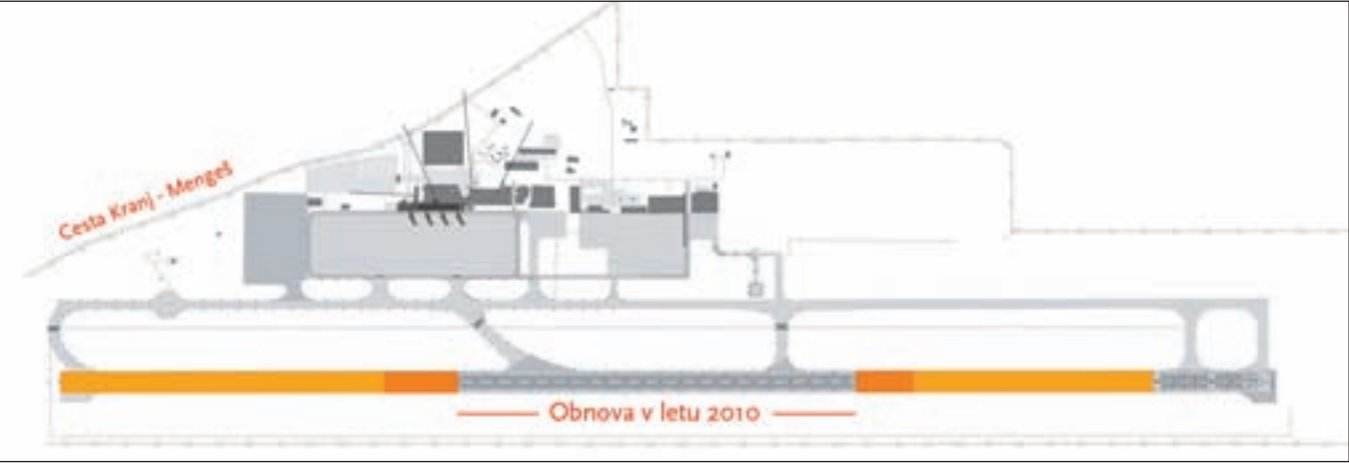
Načrt letališča na Brniku: rumeno so označeni že obnovljeni deli vzletno-pristajalne steze.
