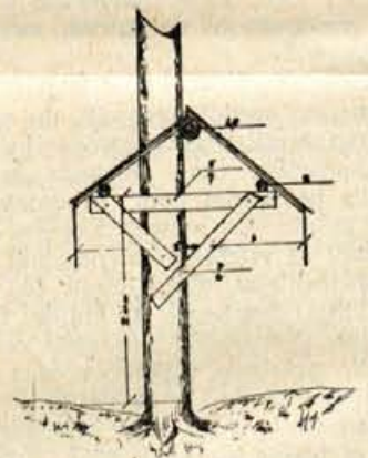
Prerez nove zaščitne strehe nad mizo in klopčama pred kurirskim bunkerjem Kokrškega odreda
