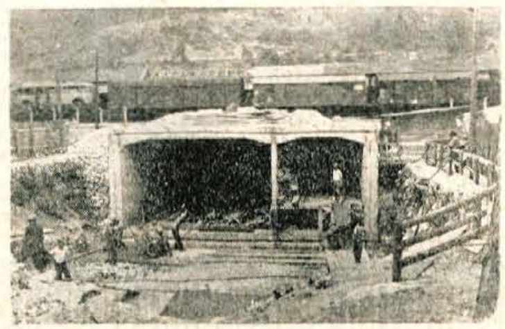
Neurejeno železniško vozlišče na Jesenicah je že vsa povojna leta velika ovira za promet, ki pa je iz leta v leto večja. Prav zaradi tega je sedaj v gradnji večji železniški podvoz (sedanji nadvoz ob hotelu Pošta, ki je bil doslej največja ovira prometu, bodo podrti), ki bo omogočil zadostno razširitev železniškega vozlišča
