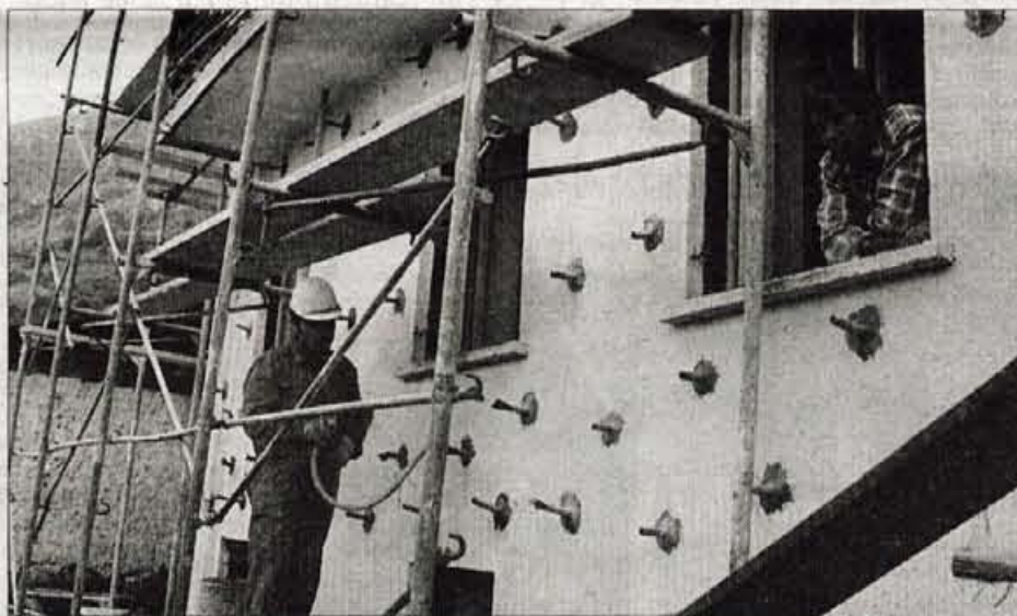
Najpogostejši način sanacije hiš, ki niso hudo poškodovane, je injiciranje betonske mase med kamenje, iz katerega so zgrajene. Utrditev temeljev in sanacija hiše na tak način stane v povprečju med 2 in 3 milijoni tolarjev.
