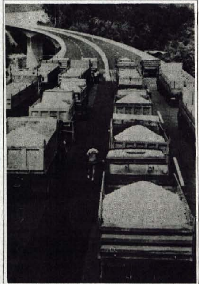
Obremenilna preizkušnja viadukta Moste - Kar tri dni je trajala obremenilna preizkušnja viadukta Moste na avtocesti Hrušica - Vrba. Osemnajst do vrha naloženih tovornjakov se je po ves dan premikalo od točke do točke, na mostu pa so merili, kako se pod težo nagiba. Taka preizkušnja je po zakonu obvezna za vse mostove, ki so višji kot 15 metrov. Viadukt Moste je bil najzahtevnejši objekt na avtocesti, saj je visok kar 72 metrov. ● D.S. - Foto: Janez Pelko
