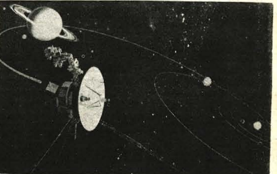
Prikaz poti ameriške sonde Voyager 1, ki je doslej poslala na Zemljo okrog 80 tisoč posnetkov, od tega 20 tisoč s Saturna, s čimer je močno okrepila dosedanje poznavanje tega zanimivega planeta.
