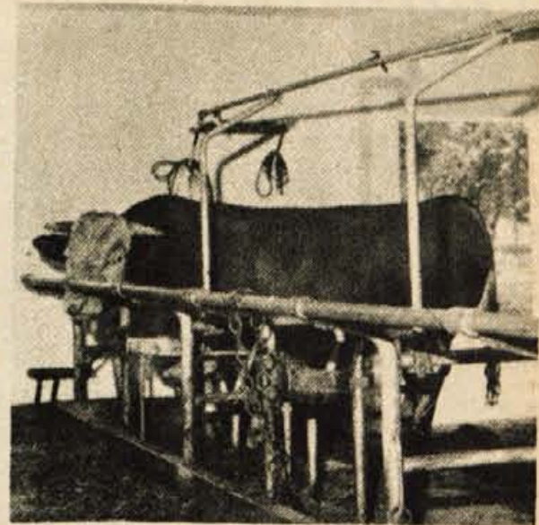
Astra TOZD Zunanja trgovina razstavlja hlevsko opremo avstrijskega izdelovalca Perchtold Johanna iz Rudena (fotografijo smo povzeli po prospektu).
