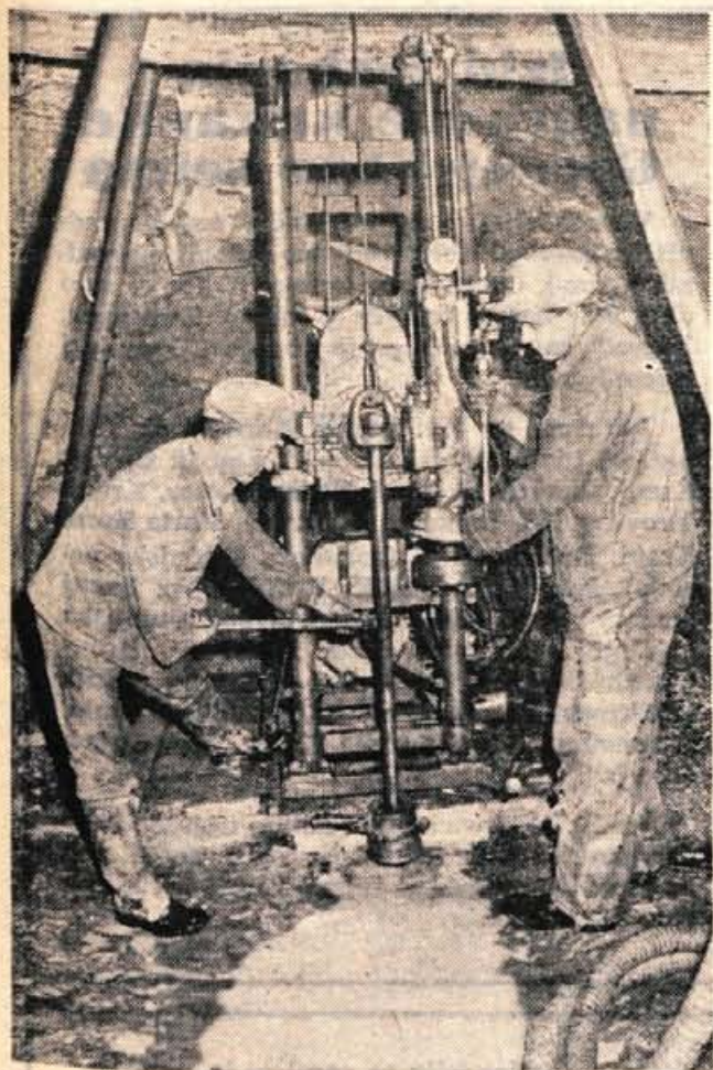
Može na koncu enega od prečnih hodnikov s posebno napravo vrtačo v tla. Odprtina ima premer le nekaj centimetrov, zato pa je zelo globoka. Iz nje dobljajo vzorce kamenin in seveda tudi delce uranove rude, če spodaj slučajno leži nova, še neodkrita plast.
