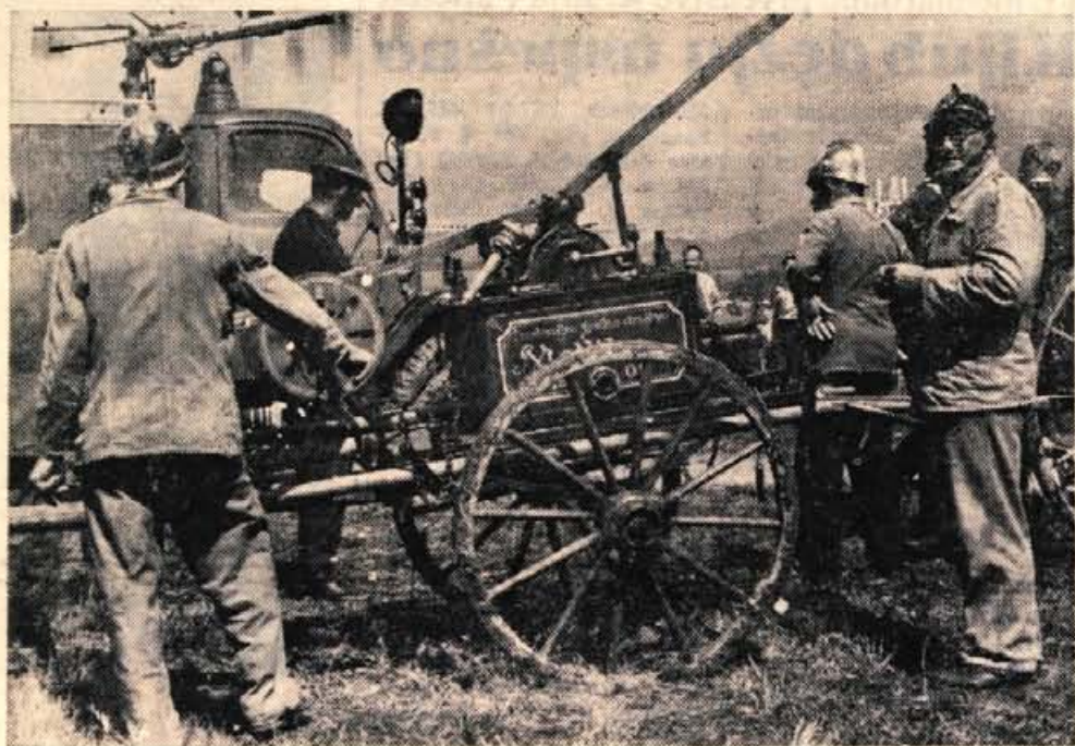
Gasilstvo nekaj in danes, bi lahko rekli za to sliko. V ospredju so metliški gasilci s šestdeset let staro črpalko, s katero pa se še vedno da gasiti. V ozadju pa je najmodernejša gasilna naprava, kar jih imamo pri nas. Na gasilnem avtomobilu je montiran vodni top za gašenje z vodo ali s peno. Top »Izstrel« 1800 litrovvode v minuti 40 metrov daleč. — Foto: S. Skrabar
